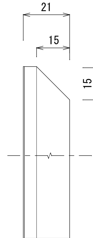
X断面詳細図
