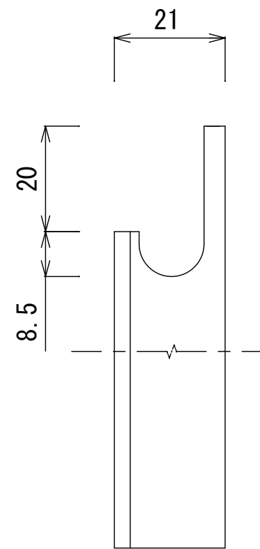
X断面詳細図
